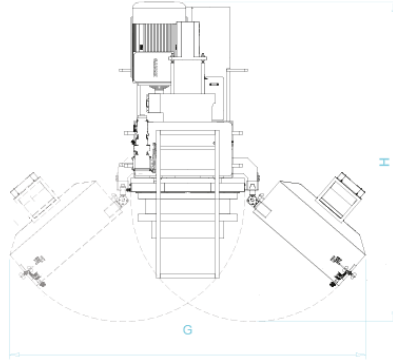
Üstten Görünüm
