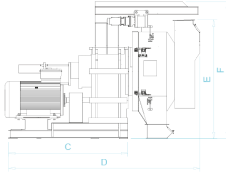
Yandan Görünüm
