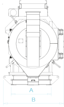
Önden Görünüm
